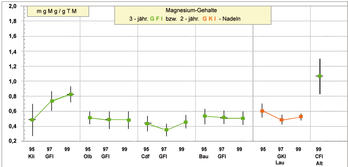
Magnesium- Gehalte [mg Mg/g TM] in rezenten sowie älteren Nadeln/Blättern von den DBF -Beständen K lingenthal, O lbernhau, C unnersdorf, B autzen, A ltenberg (Fichte= GFI ), L außnitz (Kiefer= GKI ), C olditz (Traubeneiche= TEI ) und B ad Schandau (Rotbuche= RBU , Hainbuche= HBU ) in den Jahren 1995/97/99 (Mittelwerte mit Vertrauensintervall für \alpha = < 0,05 bei n = 9 Probestämmen)
